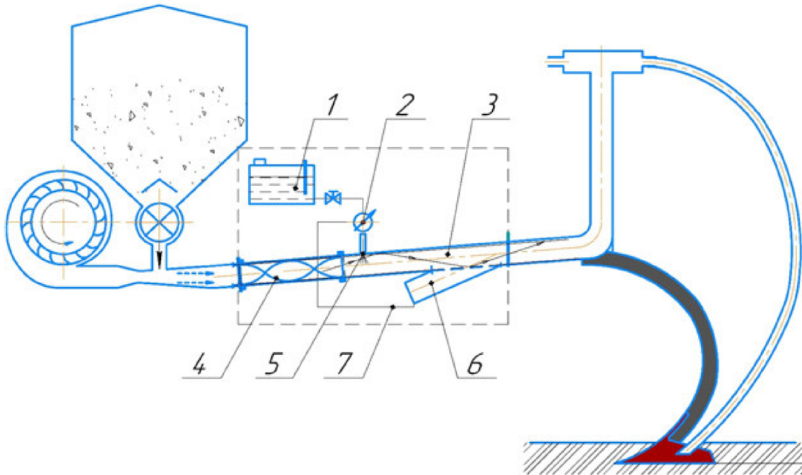
1 – емкость для рабочей жидкости; 2 – насос-дозатор; 3 – камера смешивания; 4 – винтовая поверхность (шнек); 5 – распылитель; 6 – сборник излишка рабочей жидкости; 7 – отводной патрубкок Рисунок 1 – Экспериментальный образец модуль-приставки, установленный в пневмосистему посевного агрегата
