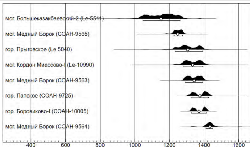
Рисунок 1 – График калиброванных дат памятников Среднего и Нижнего Притоболья первой половины II тыс. н. э.
