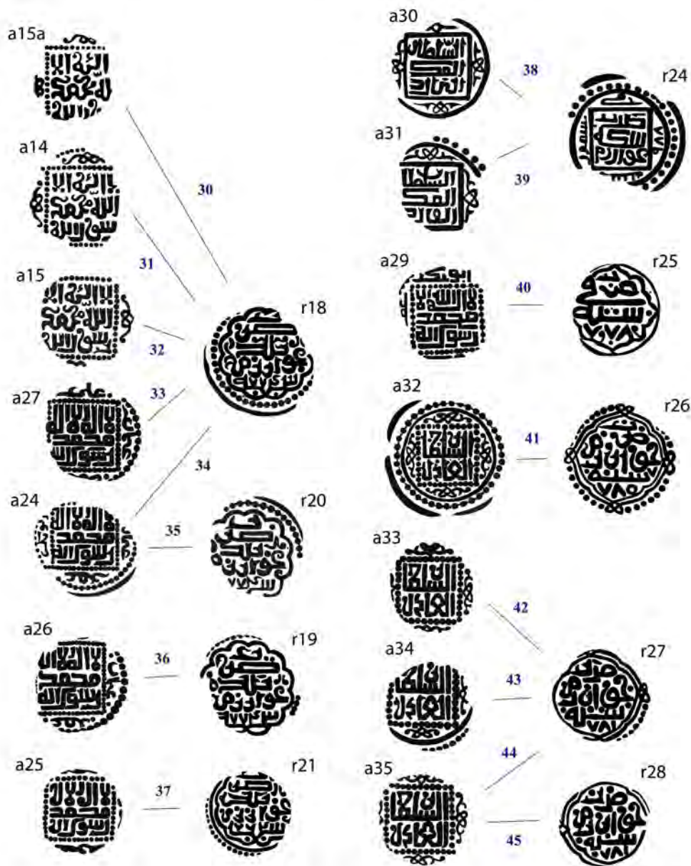
Рисунок 3 – Реконструкция итемпелей и итемпельные связи монет Хорезма
