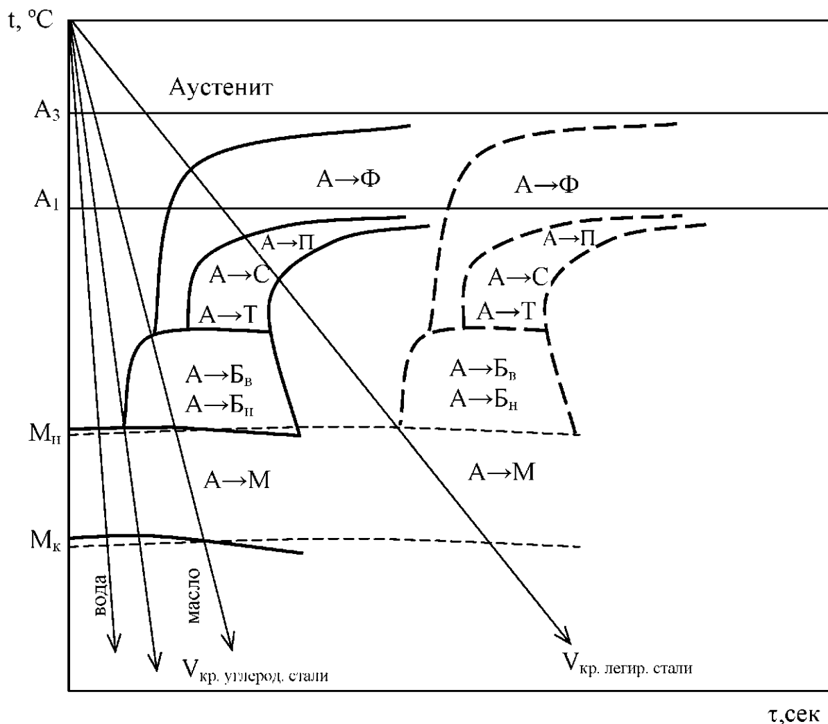
Рисунок 1 – Термокинетические диаграммы превращения переохлажденного аустенита углеродистой (сплошной линия) и легированной (пунктирная линия) сталей
