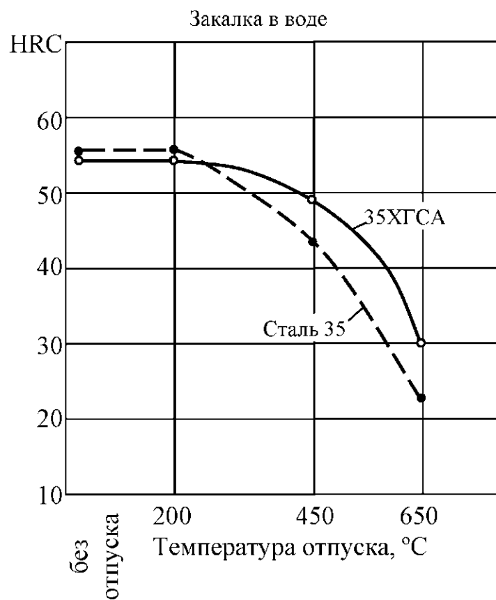
Рисунок 3 – Зависимость твердости стали от температуры отпуска после закалки в воде и масле
