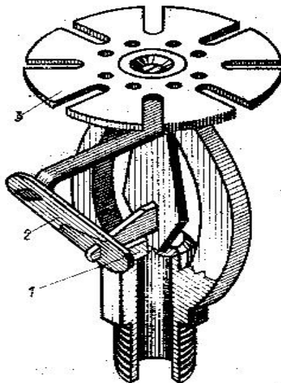
1 – клапан; 2 – замок; 3 – розетка Рисунок 6 – Спринклерная головка
