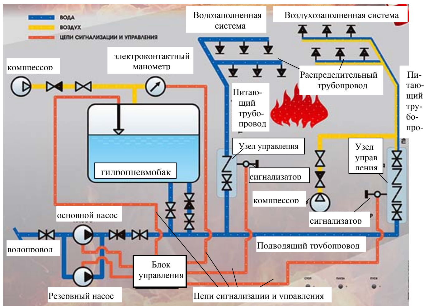
Рисунок 7 – Схема работы автоматической системы спринклерного пожаротушения
