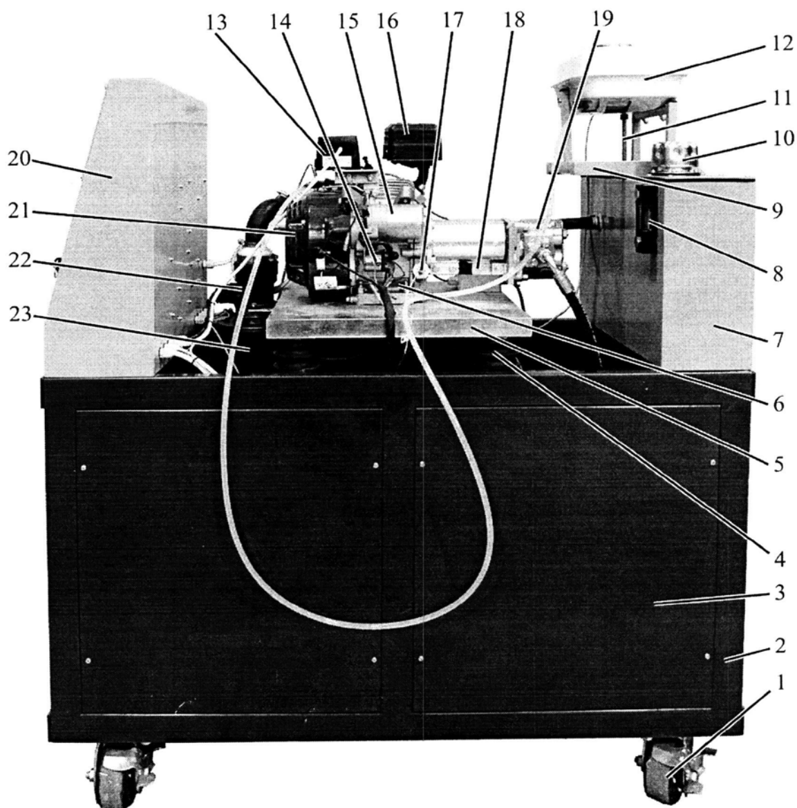
Рисунок 3.2 – Лабораторный стенд
