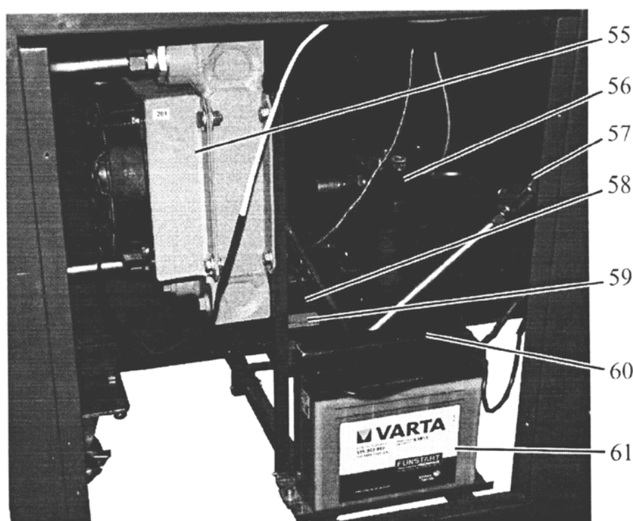
Рисунок 3.5 – Элементы гидросистемы и аккумуляторная батарея
