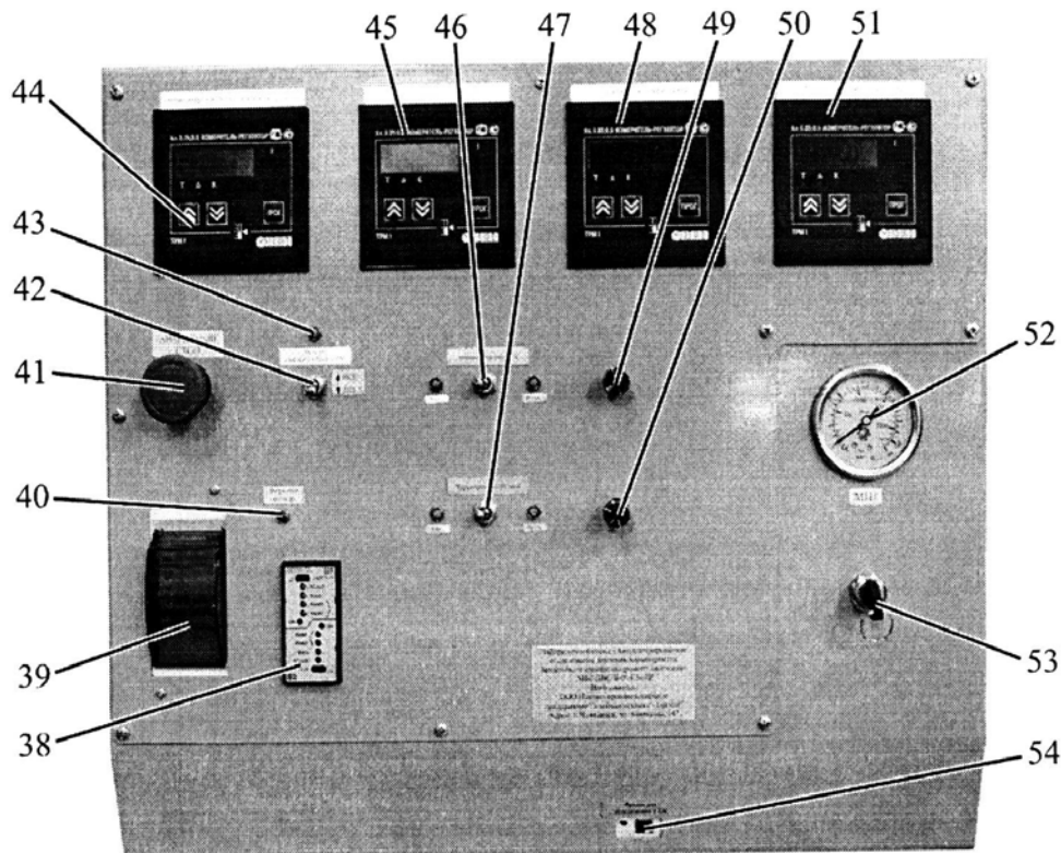
Рисунок 3.4 – Панель управления стендом
