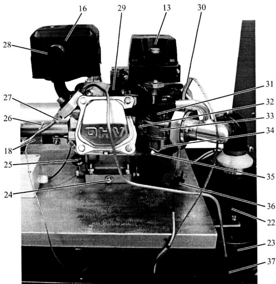
Рисунок 3.3 – Лабораторный стенд. Вид справа (фрагмент)
