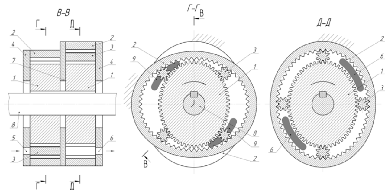
Рисунок 1 – Планетарно-роторная гидромашин
