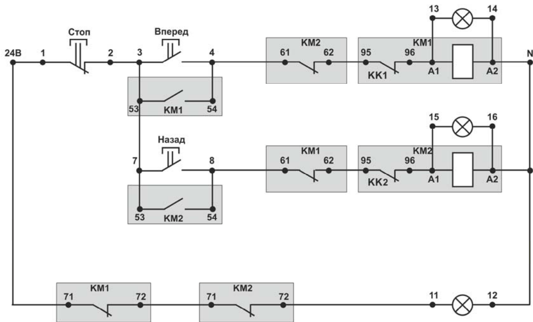
Рисунок 6 – Схема управления асинхронным двигателем с возможности реверса
