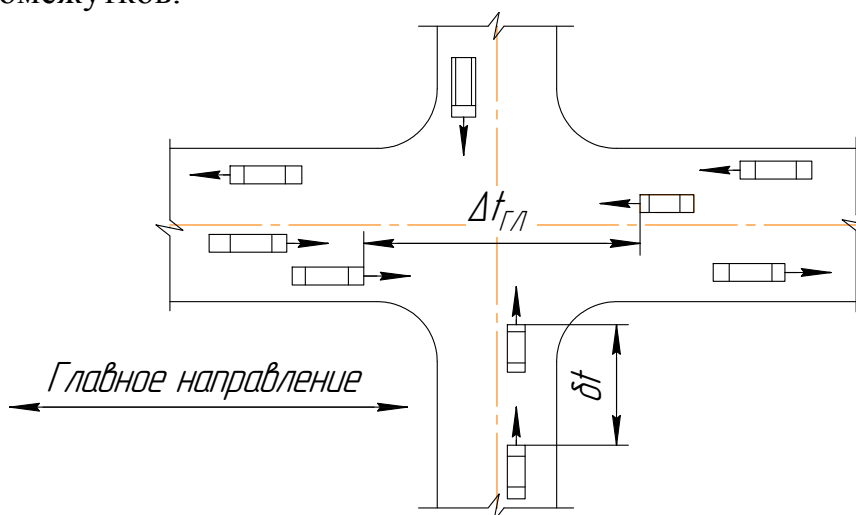
Рисунок 3.1 - Расчетная схема
