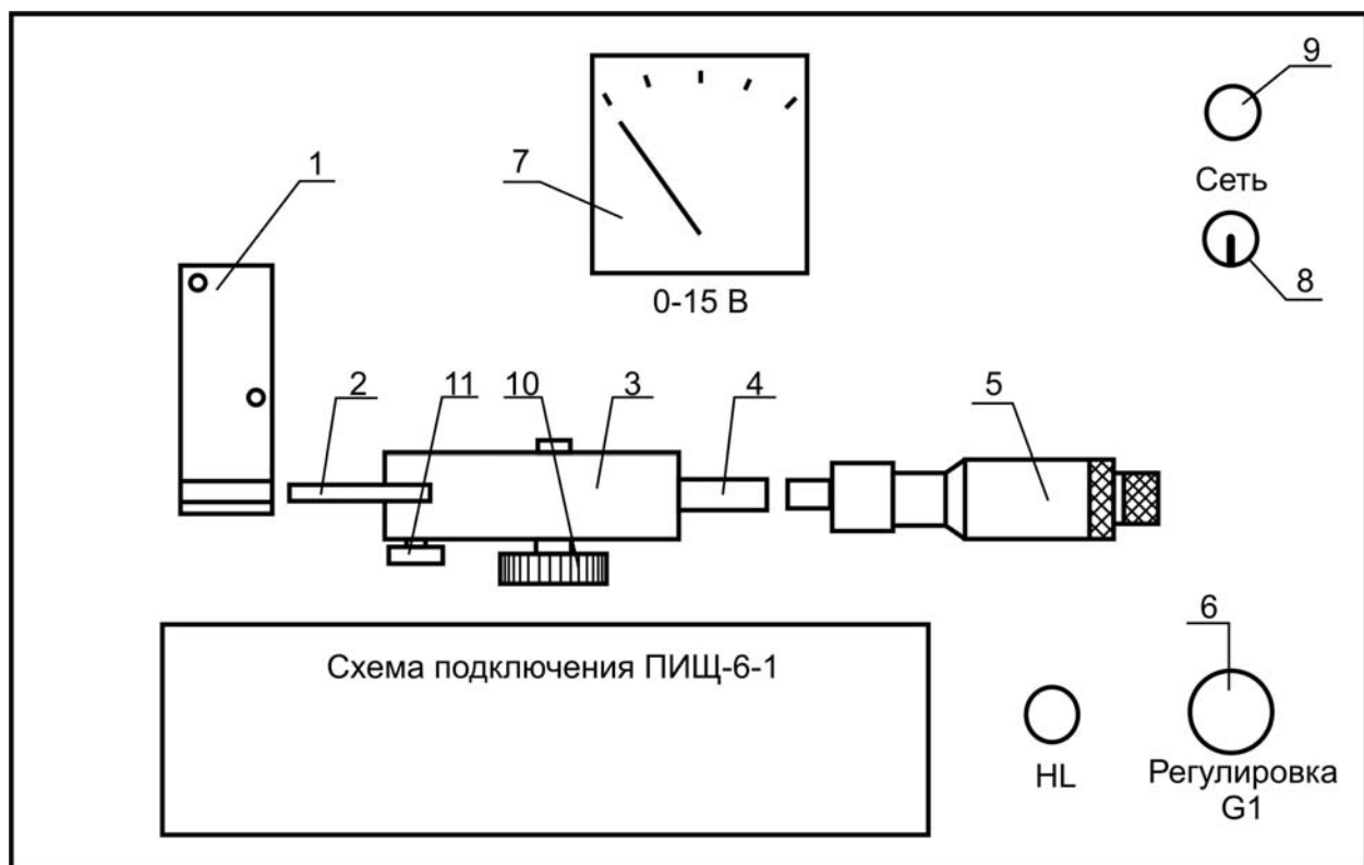
Рисунок 6 – Общий вид передней панели станда
