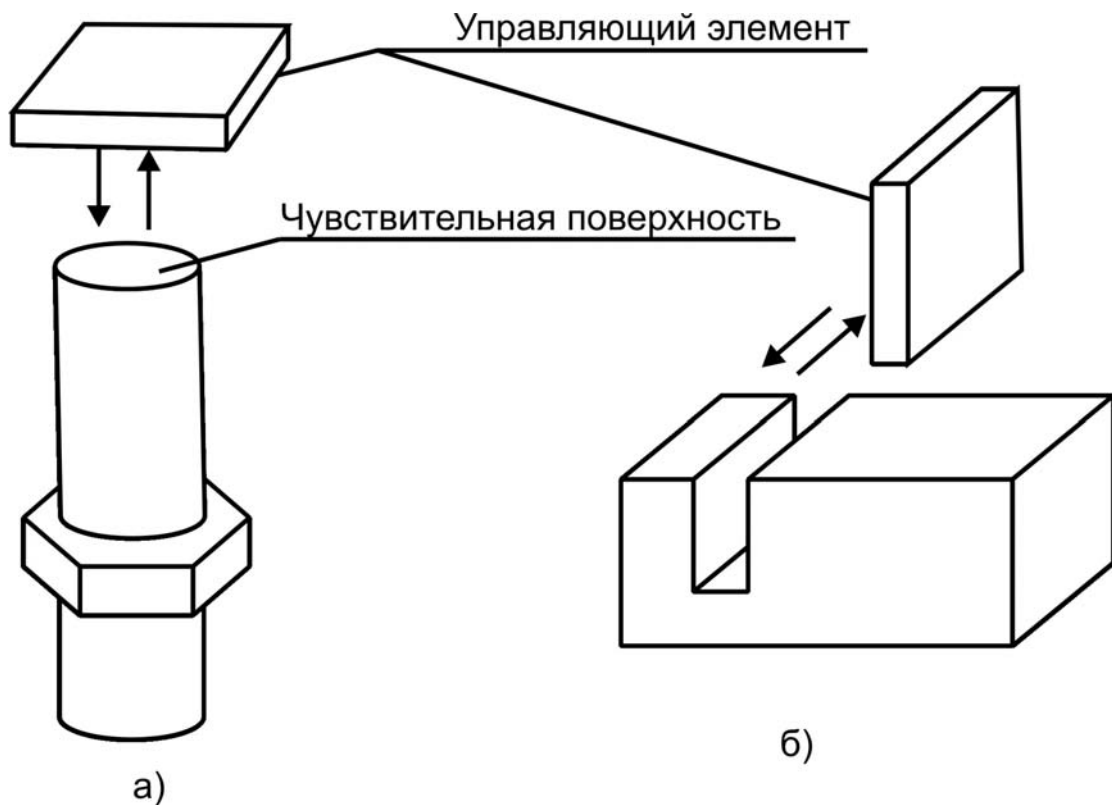
Рисунок 2 – Конструктивное исполнение индуктивных путевых выключателей
