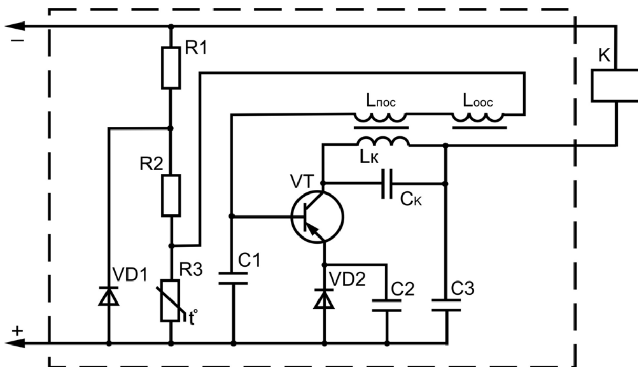
Рисунок 4 - Электрическая принципиальная схема путевого выключателя
