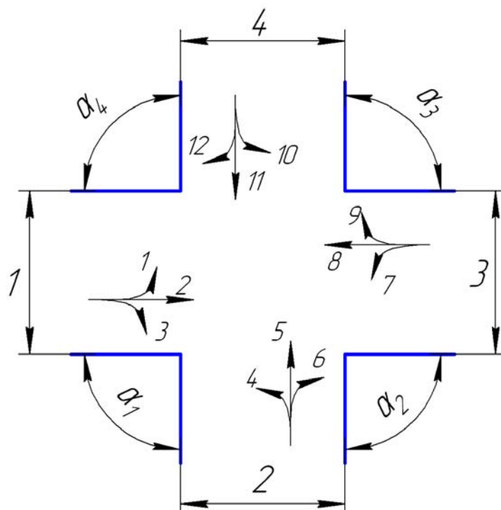
Рисунок 2.1 - Схема перекрестка и условные обозначения
