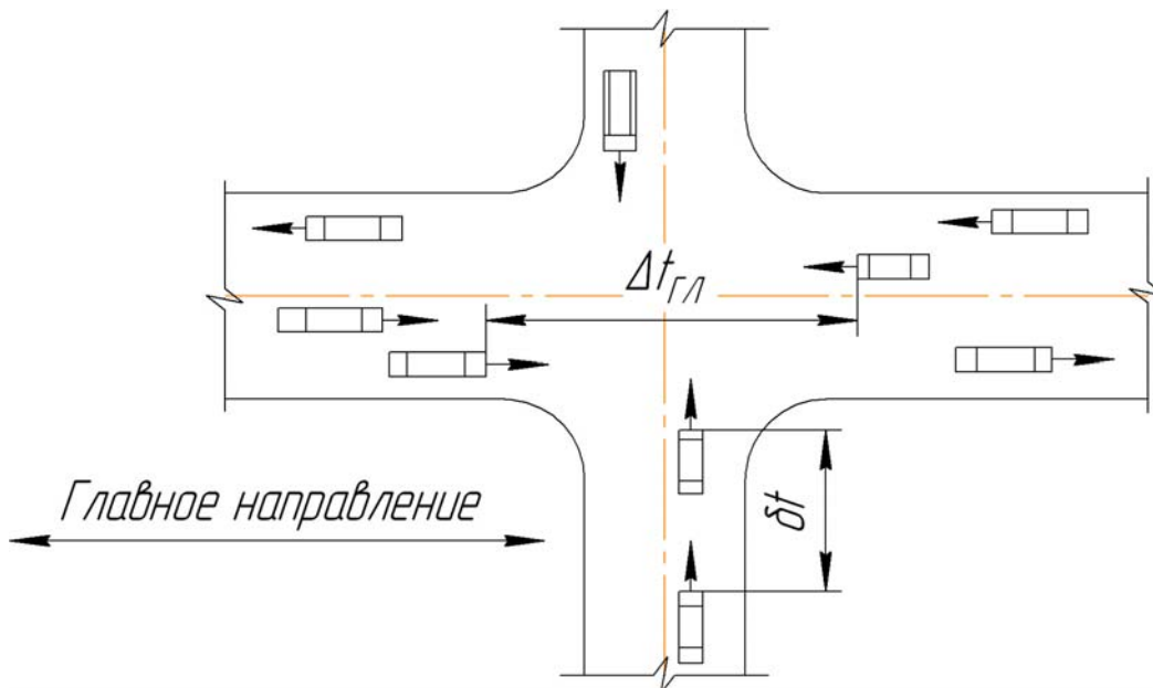
Рисунок 3.3 - Расчетная схема
