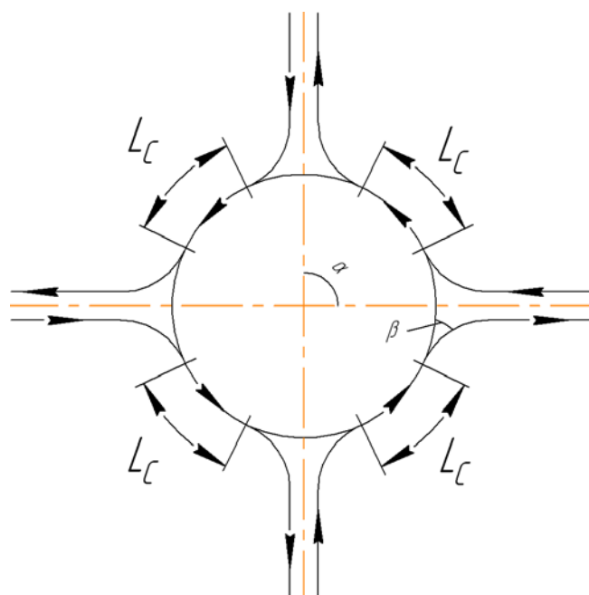
Рисунок3.5- Геометрическая схема кольцевого саморегулируемого узла
