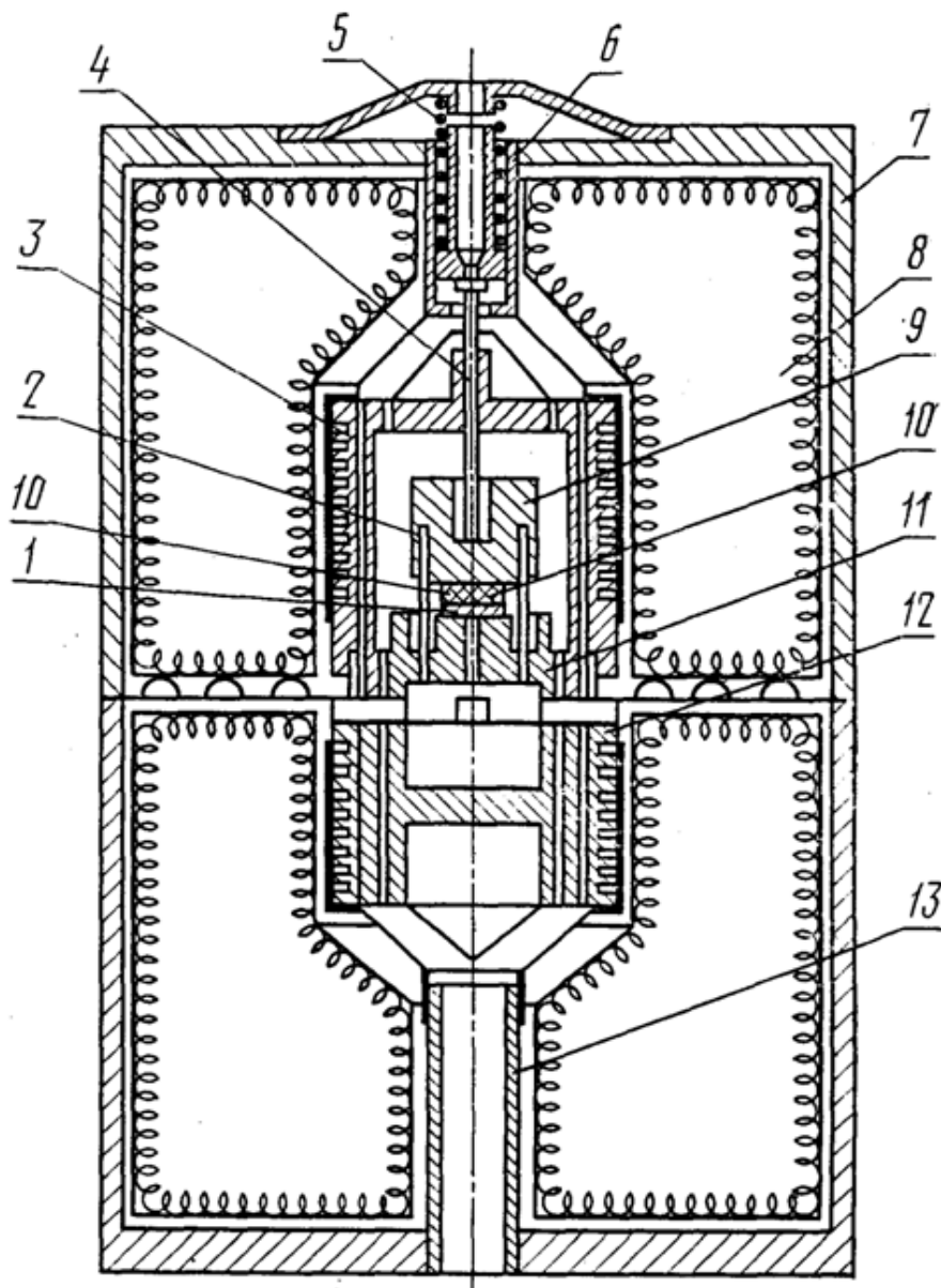
Рис. 2. Измерительная ячейка
