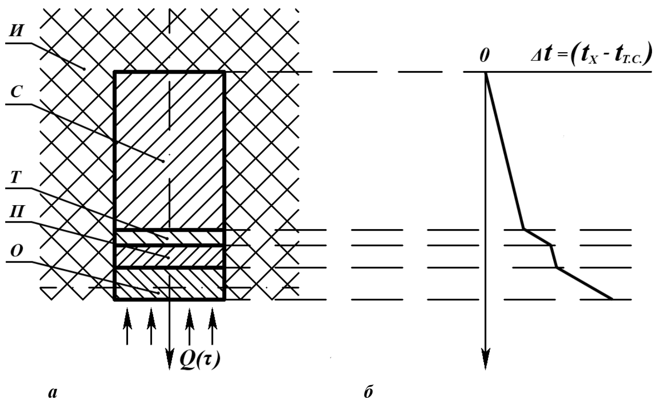
Рис. 1. Тепловая схема метода
